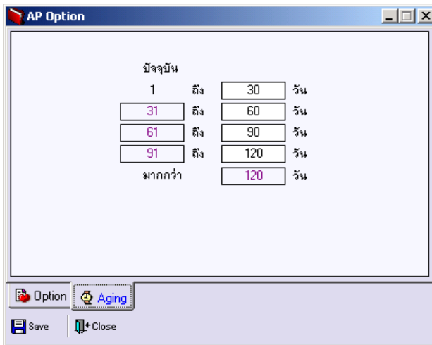
ตัวอย่างการกำหนด AP Option Tab Aging
